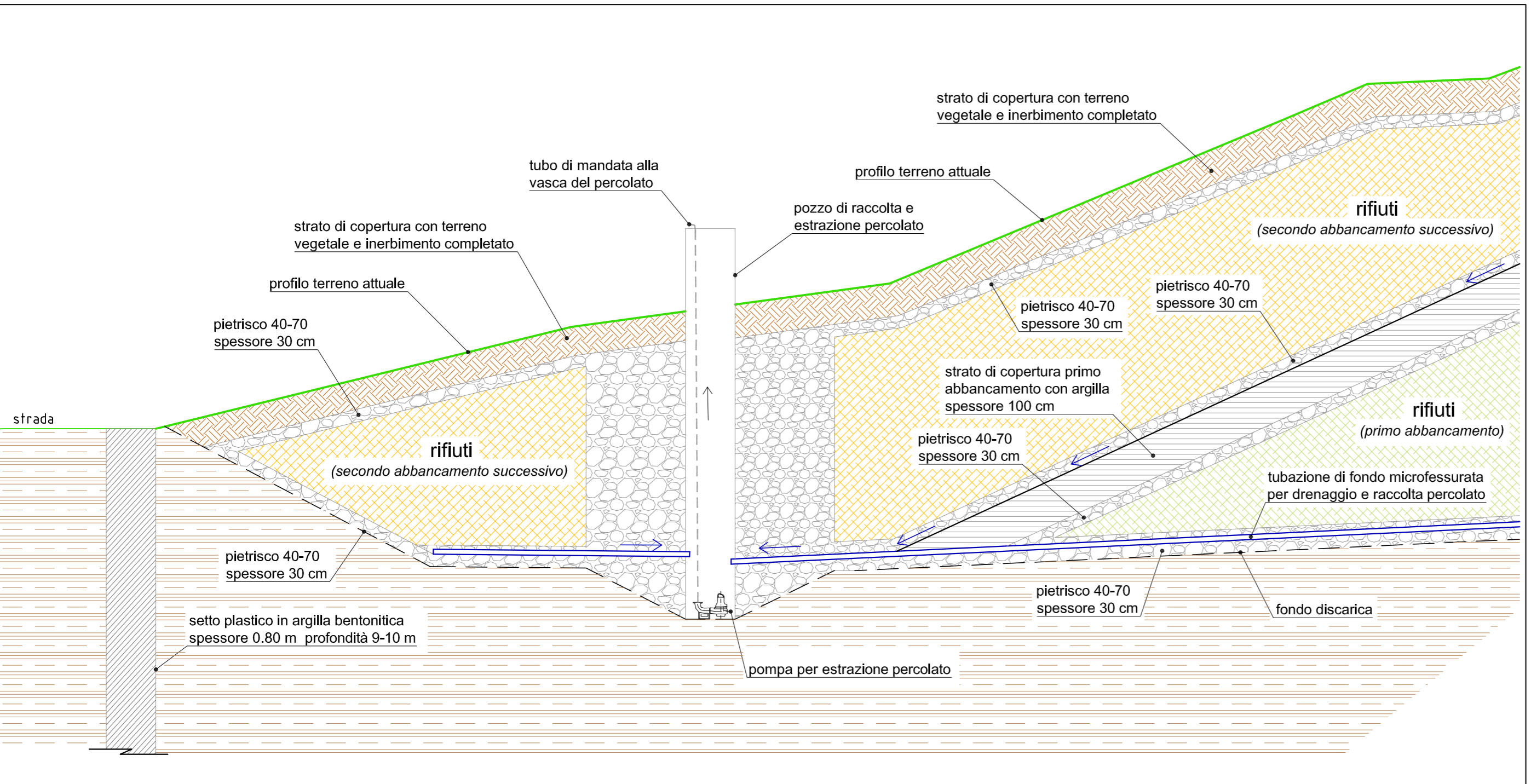
PARTICOLARE 1: SCHEMA DEL SISTEMA DI RACCOLTA ED ESTRAZIONE DEL PERCOLATO - scala 1:100
