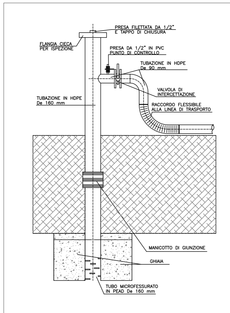
PARTICOLARE TESTA POZZO - scala 1:20
