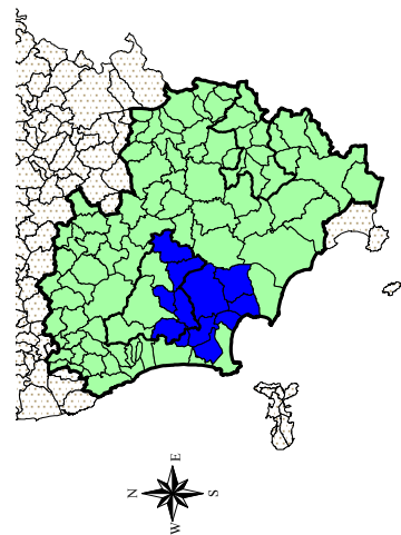
Figura 6.1.43 - Cluster significativi, periodo 2000-2006, rif. area 50 km.
